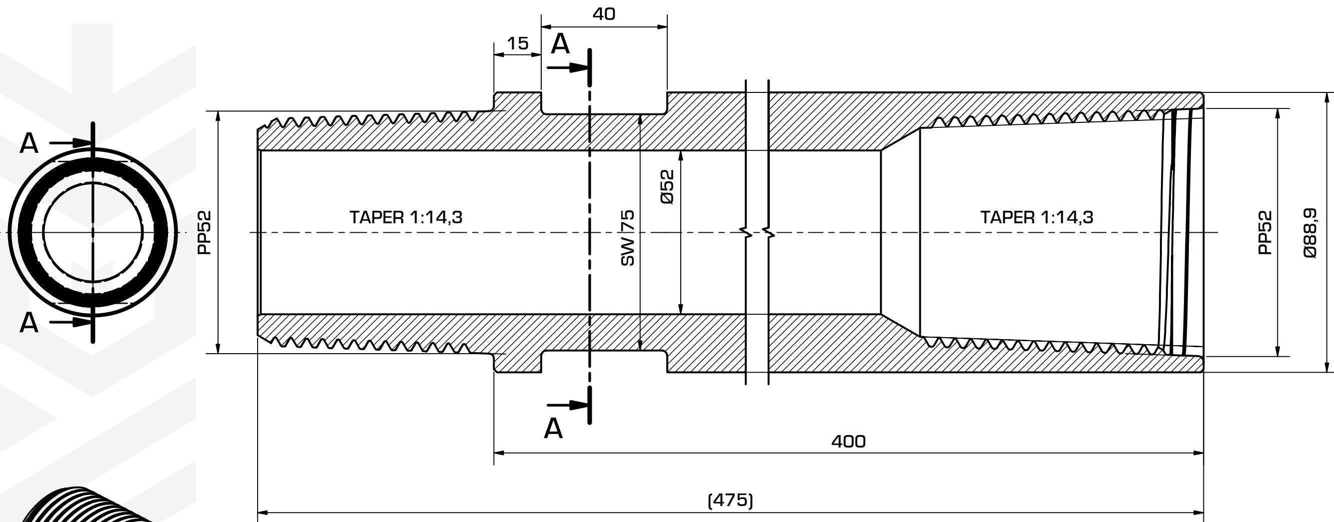
A-A (1:2)
